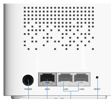
Power Input WAN LAN 1-2 Reset
